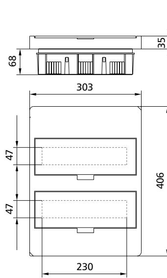
BC-U-2/24(-TW)-ECO
