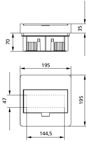
BC-U-1/8(-TW)-ECO
