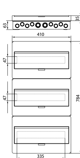
BC-O-3/54(-TW)-ECO
