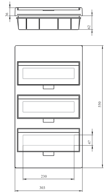
BC-U-2/36(-TW)-ECO
