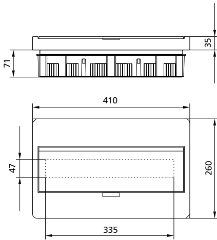
BC-U-1/18(-TW)-ECO
