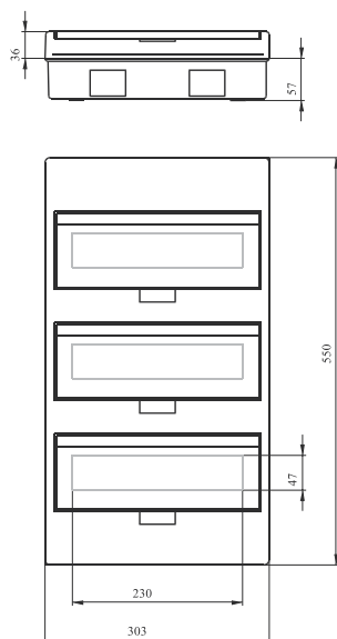
BC-O-3/36(-TW)-ECO
