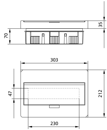
BC-U-1/12(-TW)-ECO
