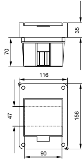
BC-U-1/5(-TW)-ECO
